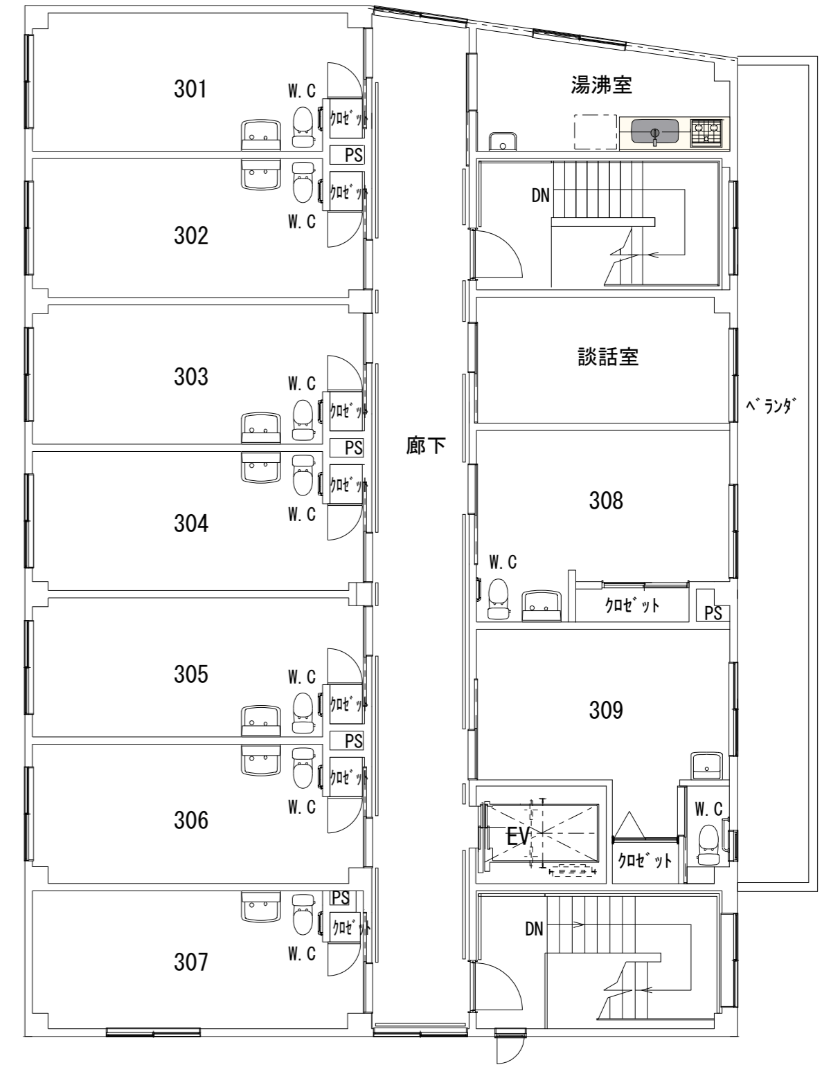
3階平面図
