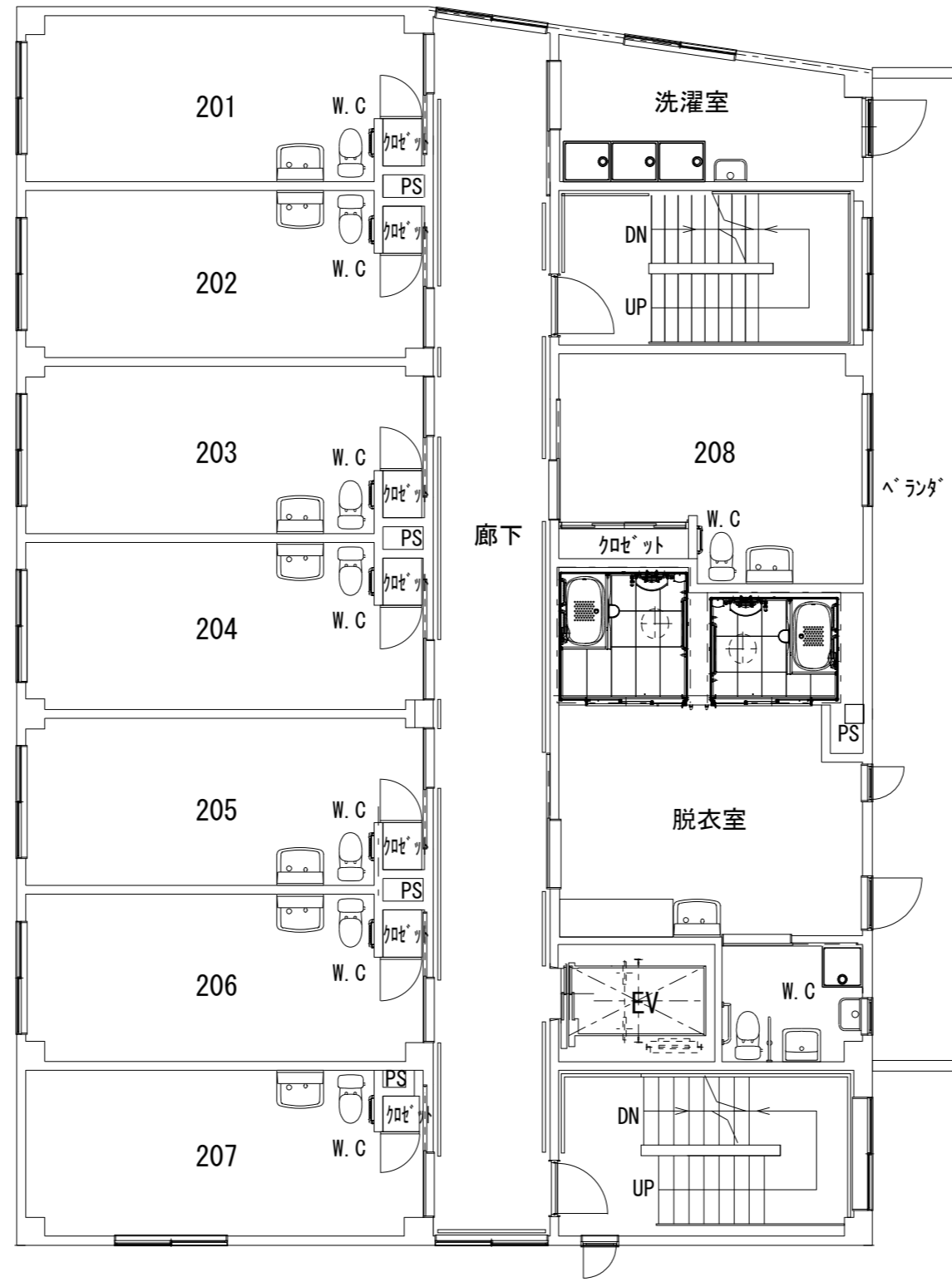
2階平面図
