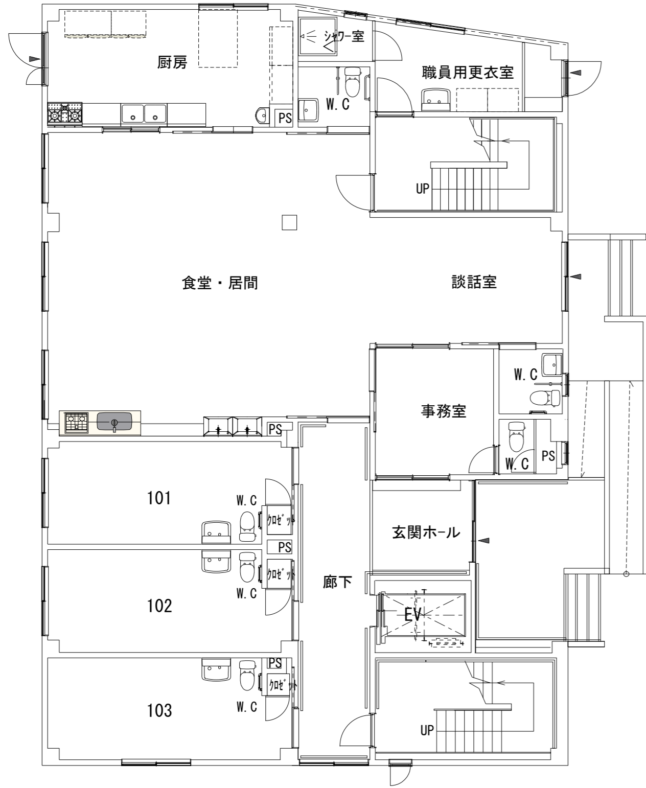
1階平面図
